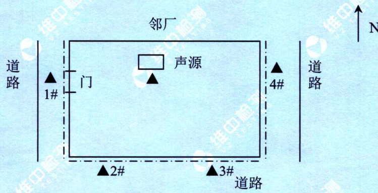
附: 工业企业厂界环境噪声检测点位示意图
